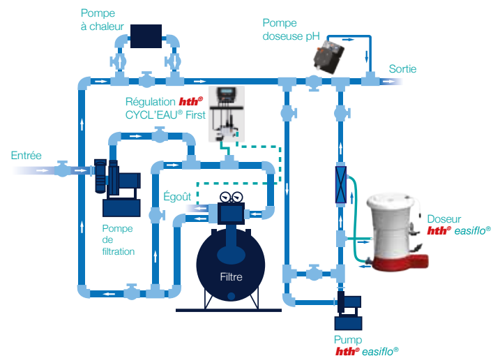
Shéma d'installation type régulation hth ® CYCL'EAU® First avec doseur hth ® easiflo® First
